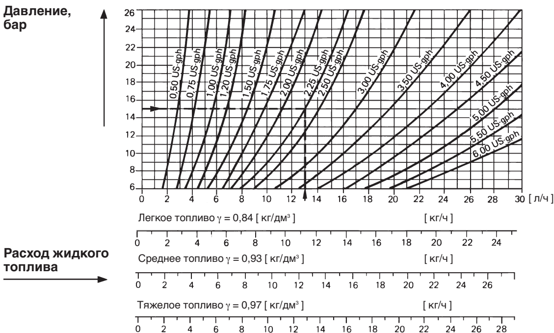
Диаграмма подбора форсунок Simplex
