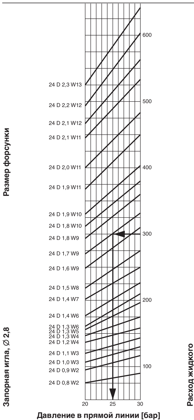
Диаграмма подбора форсунок, тип 24 Форсуночный блок MDK70
