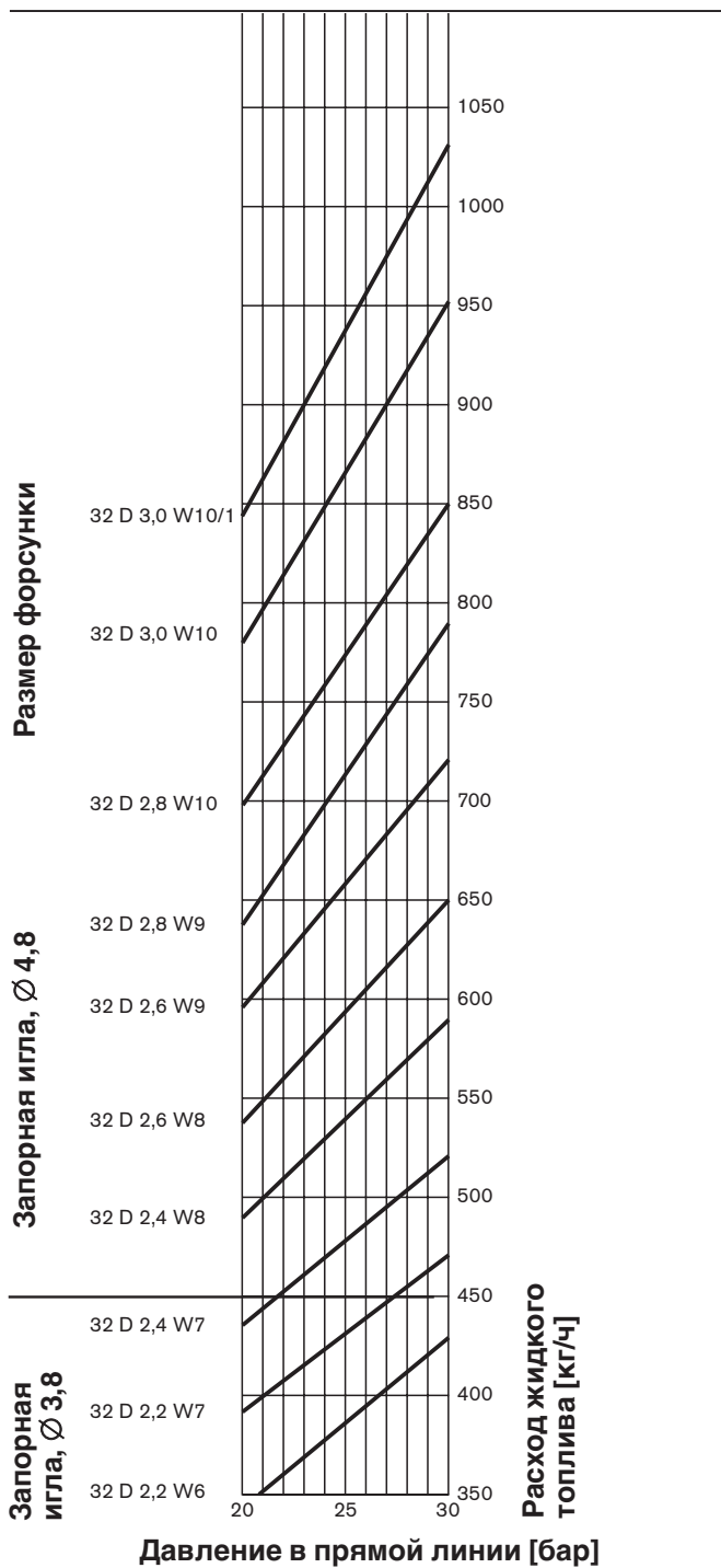
Диаграмма подбора форсунок, тип 32 Форсуночный блок MDK80
