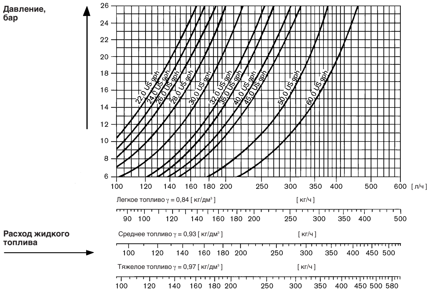
Диаграмма подбора форсунок Simplex
